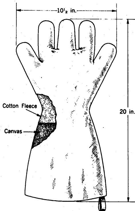
Fig. 7 - Asbestos Glove
