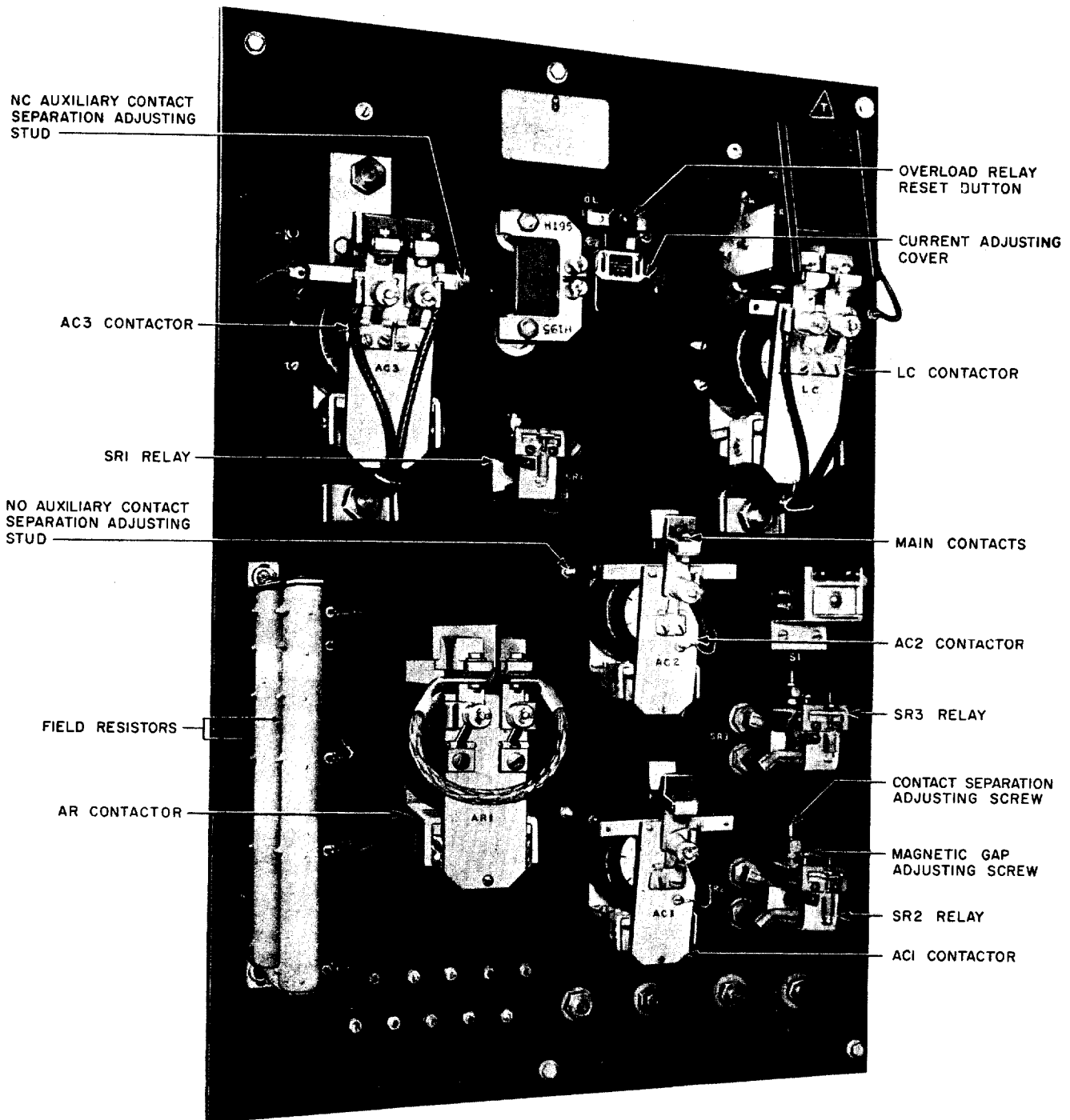
Fig. 6 - KS-15582 L5 Starter
