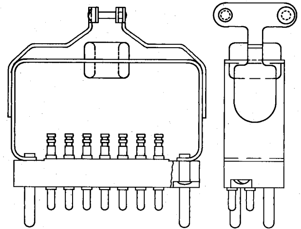
Fig. 14—KS-16322 Connector
