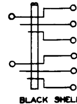
Fig. 2—211, 212, or 213 Plug
