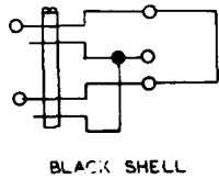
Fig. 18—241C Plug
