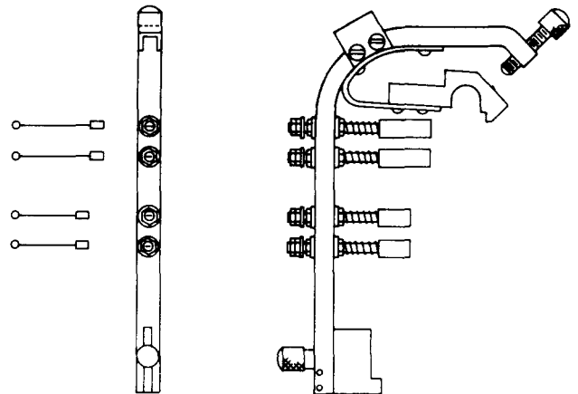
Fig. 22—243 Plug
