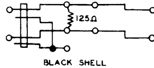
Fig. 7—381A Plug
