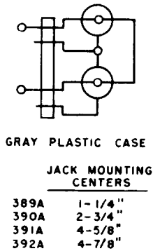
Fig. 13—389A, 390A, 391A, or 392A Plug
