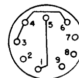
Fig. 3—377A Plug
