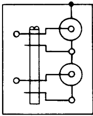
Fig. 5—379A Plug
