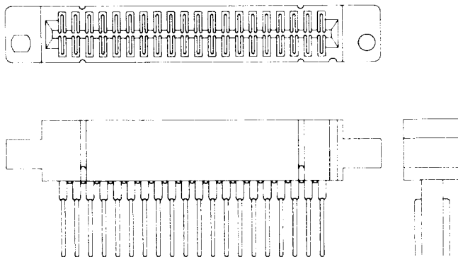
Fig. 11—928A, D, or E Connector
