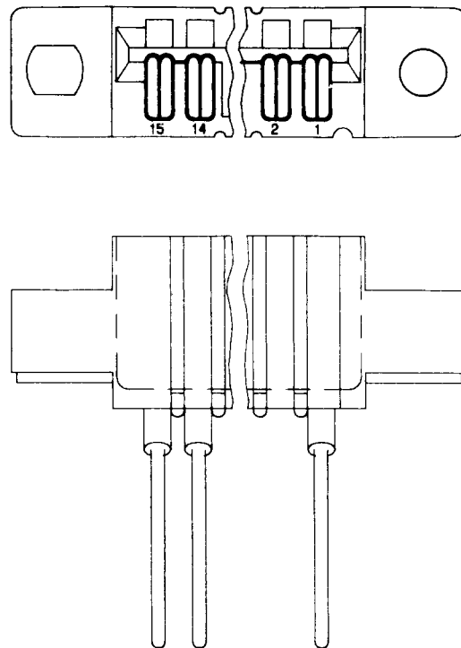
Fig. 18—935A Connector
