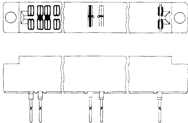
Fig. 14—931A, C, E1, E2, or E3 Connector
