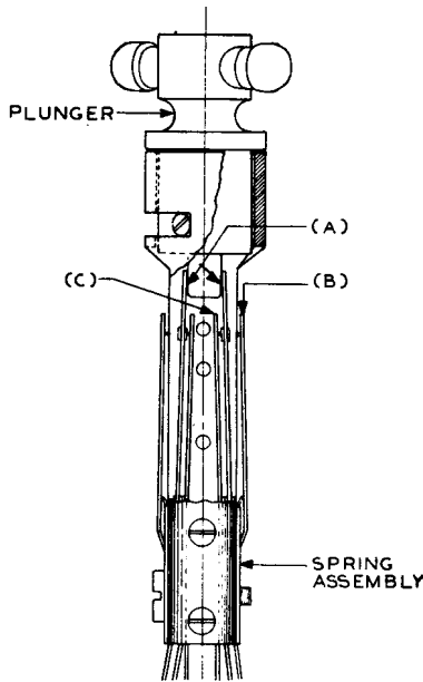
Fig. 6 - 272-type Key
