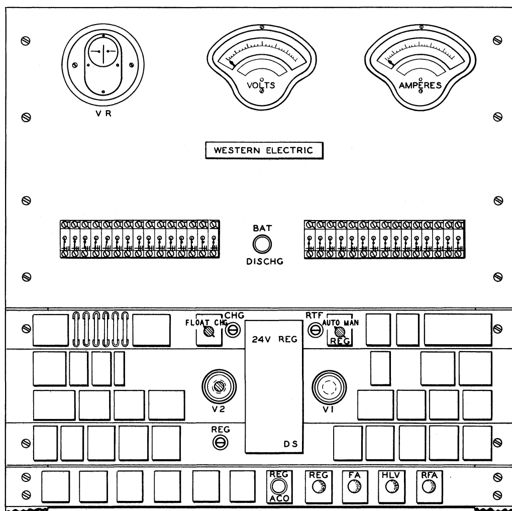
Fig. 3—110A 24-Volt Plant Controls
