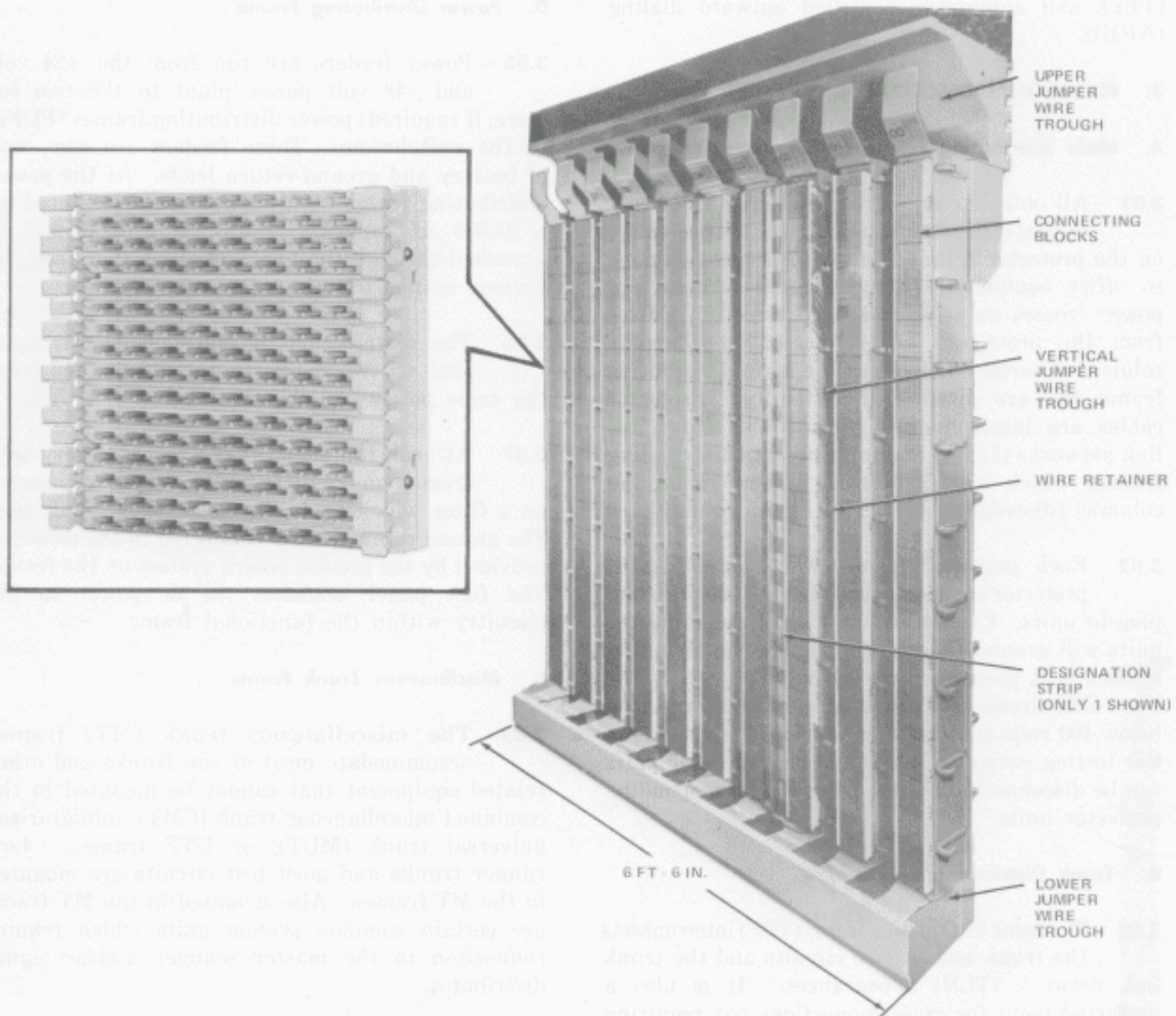
Fig. 1—Main Distributing Frame Module
