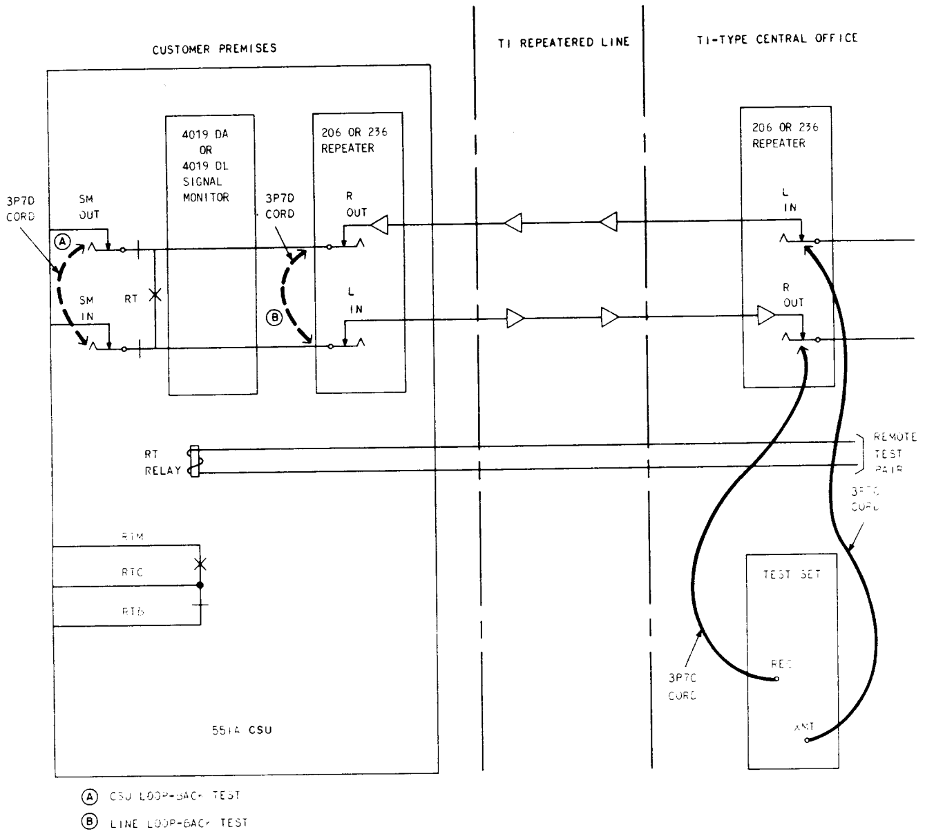
Fig. 1—Remote Loopback Test
