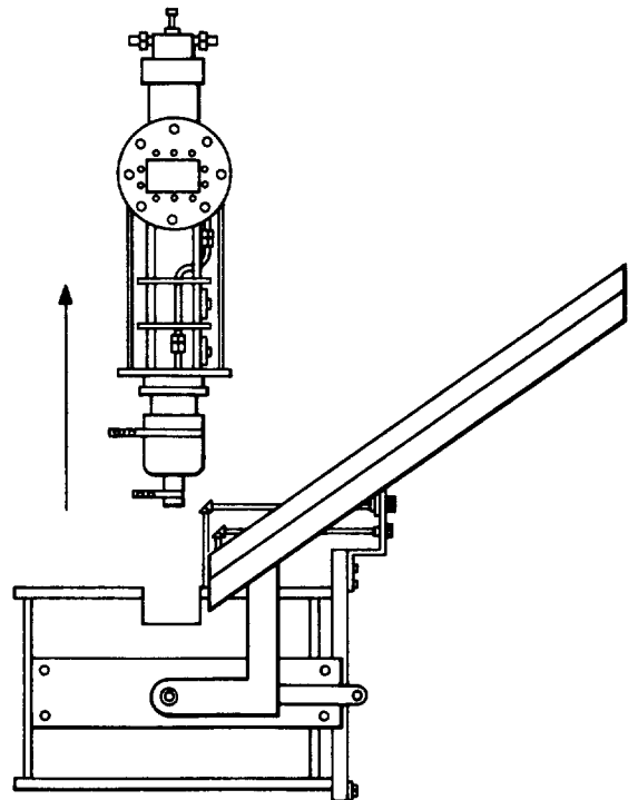
D-KLYSTRON REMOVAL
