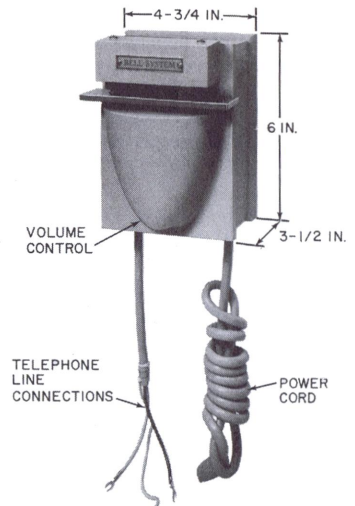
Fig. 14—KS-8229 Chime
