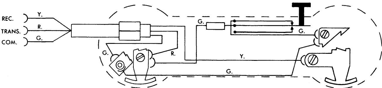
3A. Type 84 Handset
