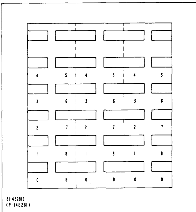
Fig. 5—811452812 (P-14E281) Designation Strip
