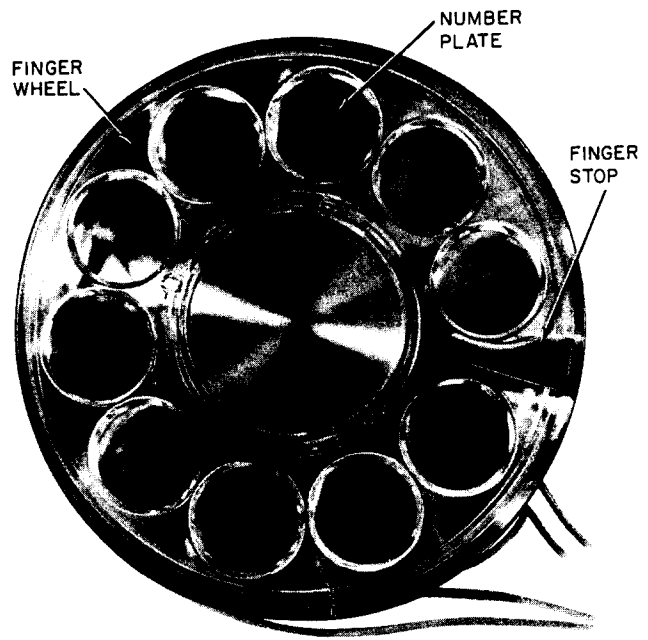
Fig. 5—11E Dial, Front View
