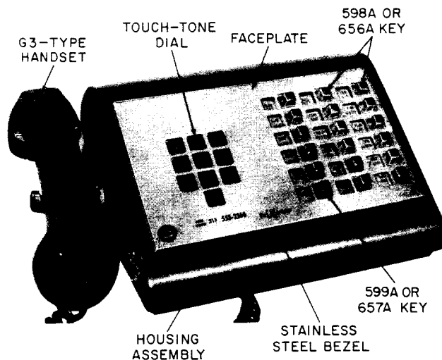
Fig. 1—1630-Type Telephone Set
