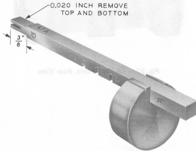
Fig. 21 – 147A Gauge
