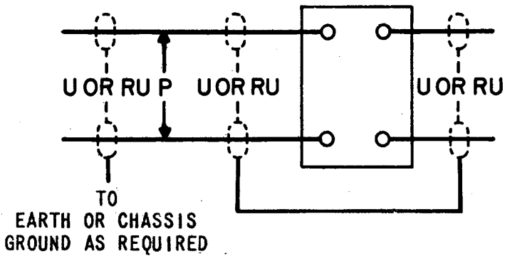
(d) Typical paired and shielded wiring
