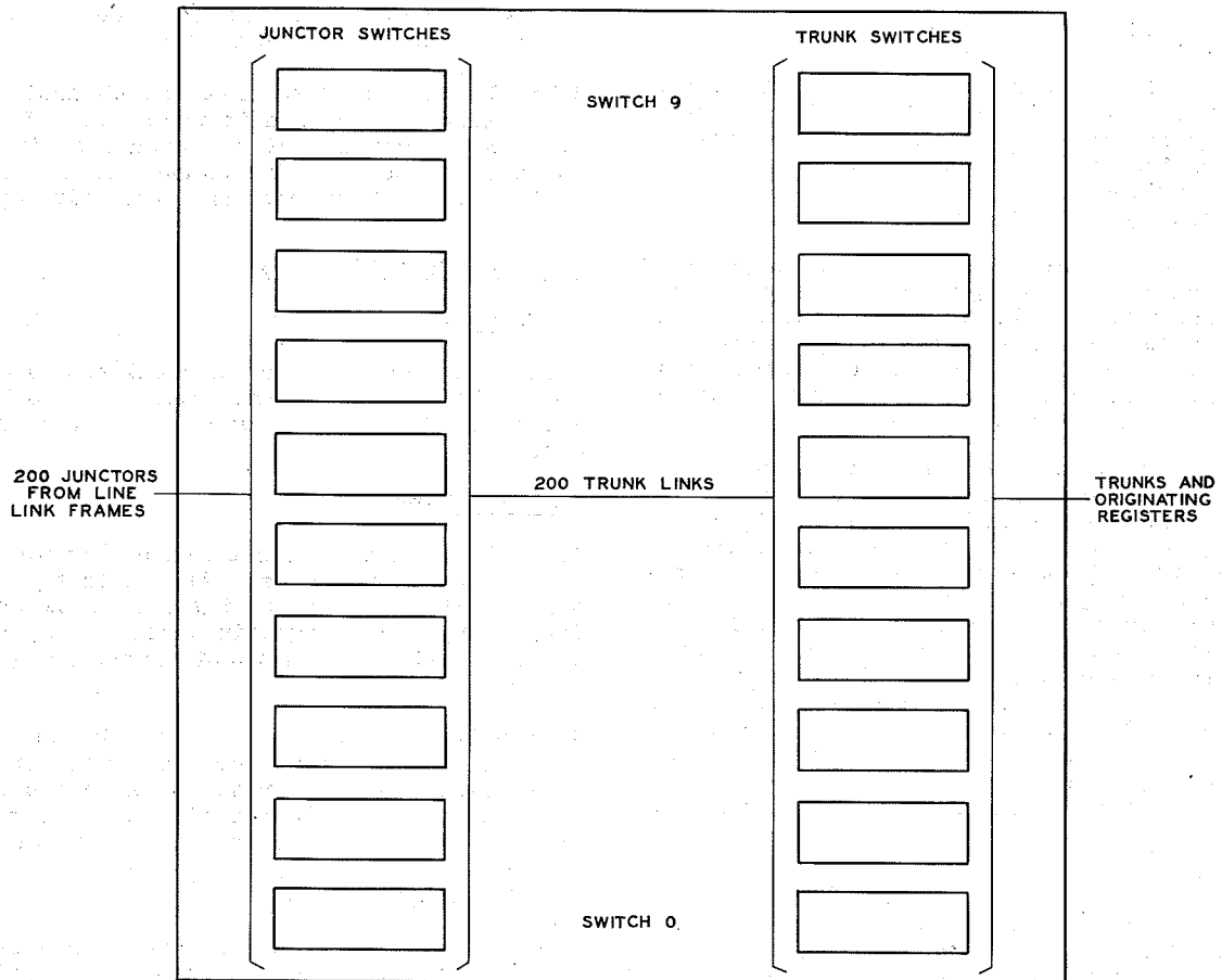
Fig. 7 - Trunk Link Frame
